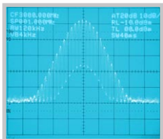
Signal 3 GHz Modulé en amplitude
